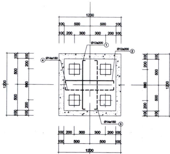
ĐAI MÓNG MC1 (TL:1/20)
