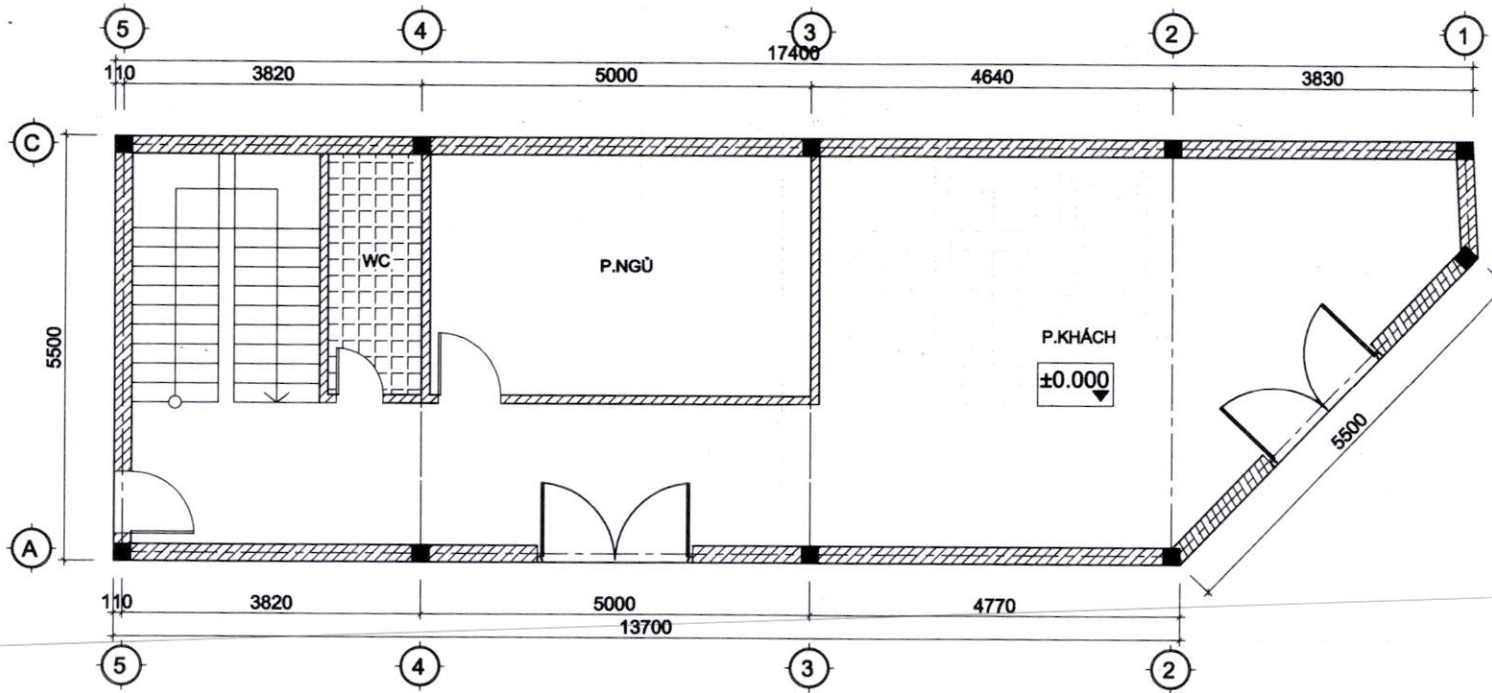
MẶT BẰNG TẦNG 1
