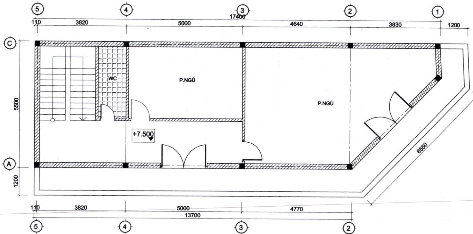
MẶT BẰNG TẦNG 3
