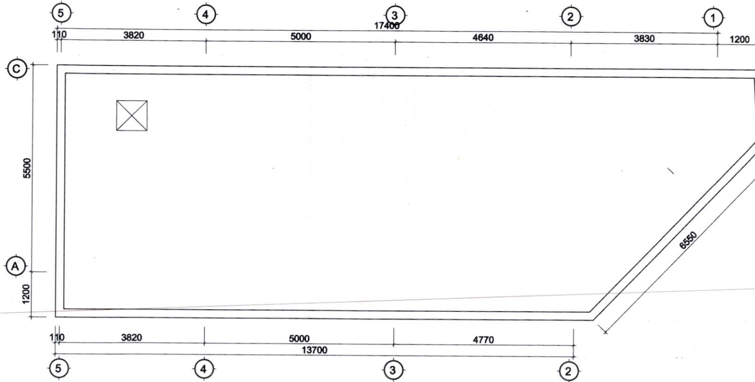
MẶT BẰNG MÁI
