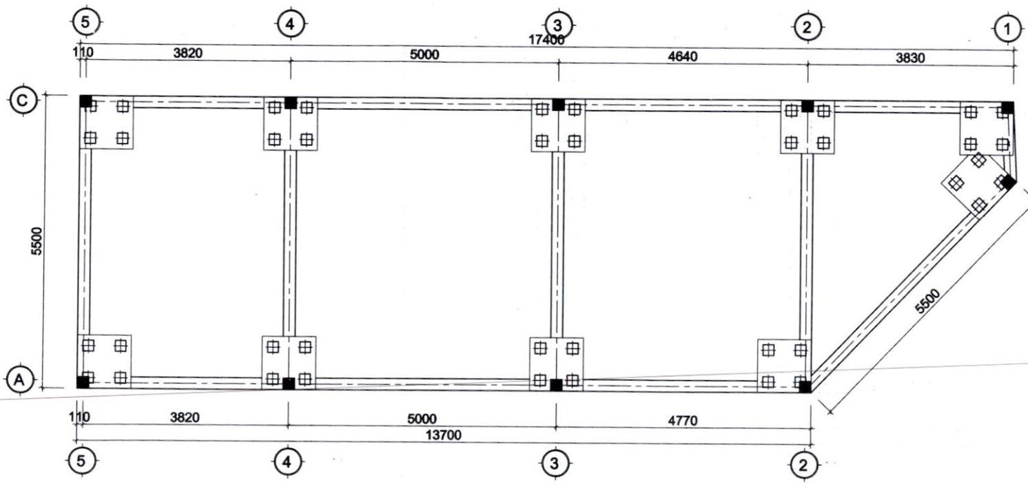
MẶT BẰNG MÓNG
