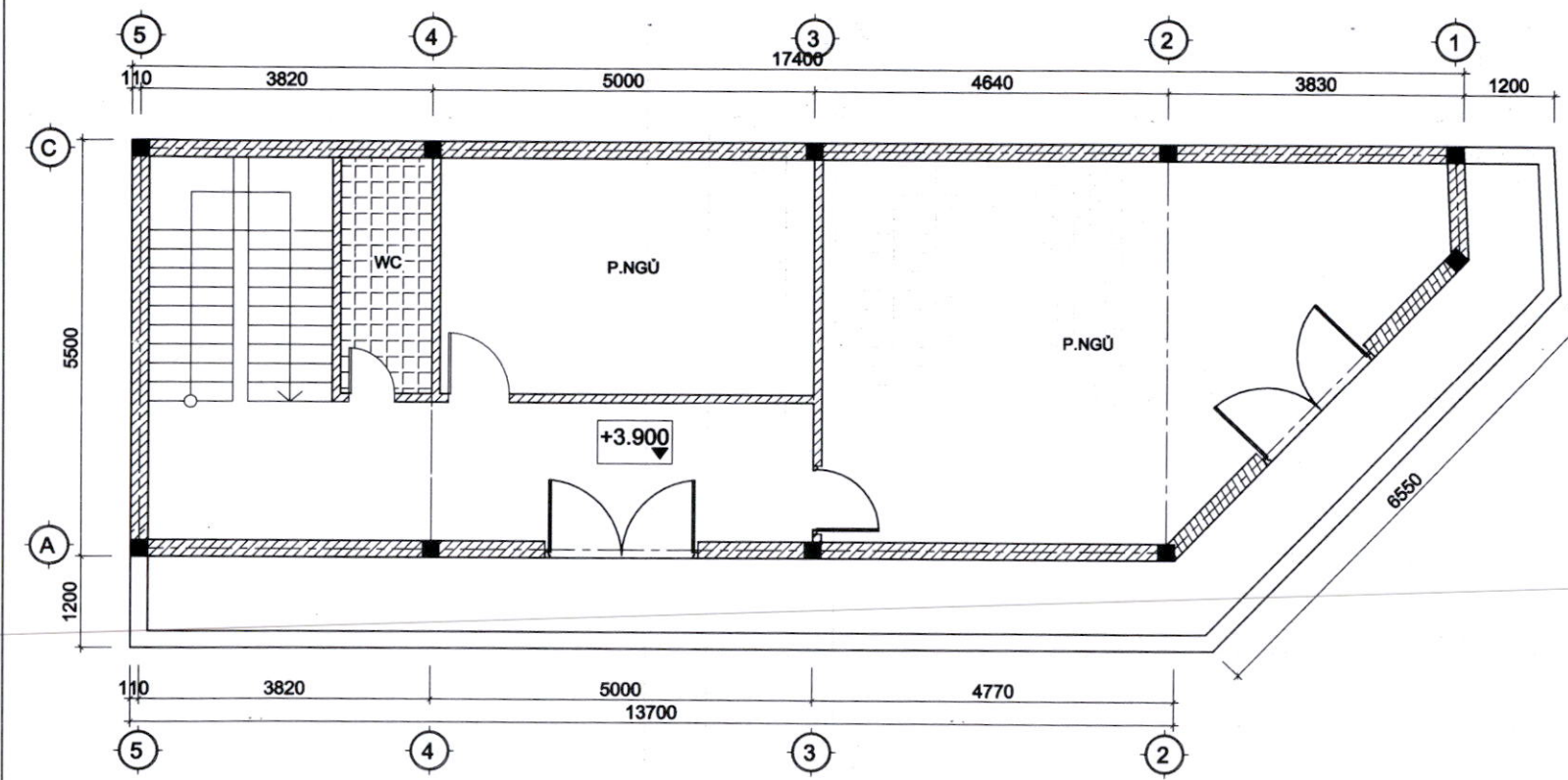
MẶT BẰNG TẦNG 2
