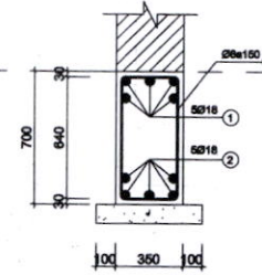
DÀM MÓNG DM1
